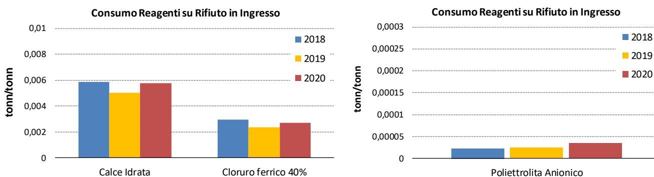
Figura 18 Andamento dell'indicatore "Fattore di utilizzo reagenti"
