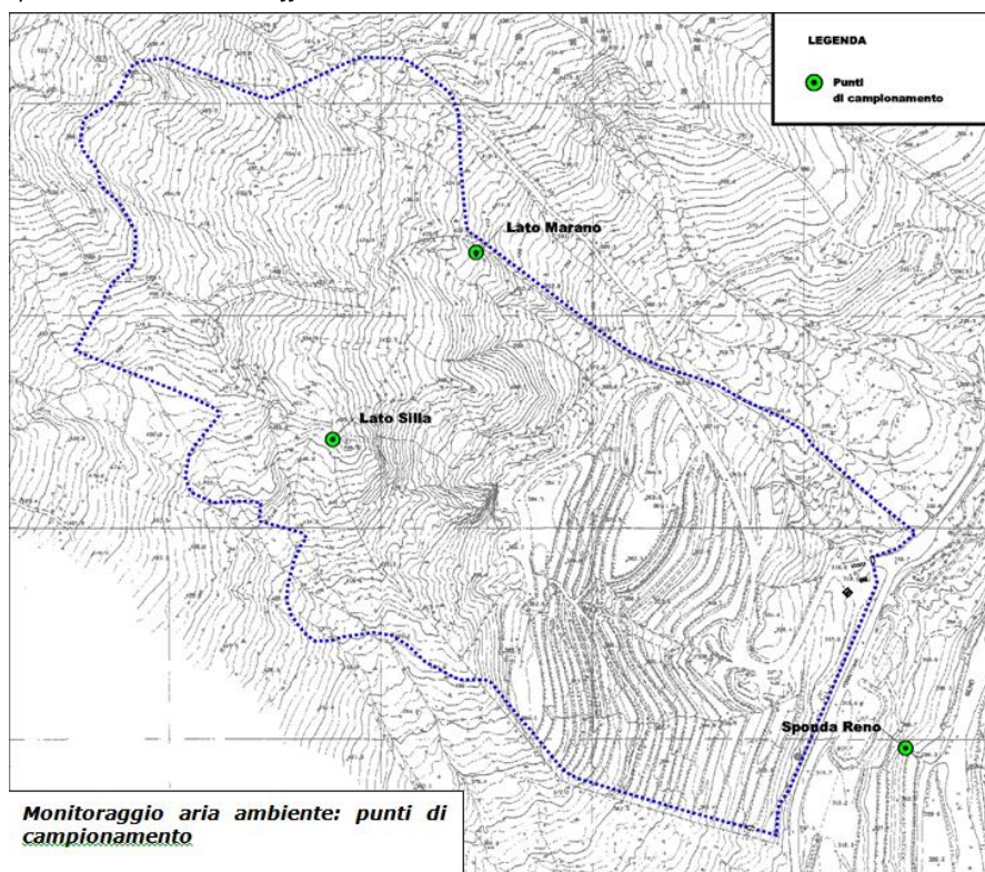
Figura 18 Punti di campionamento emissioni diffuse
