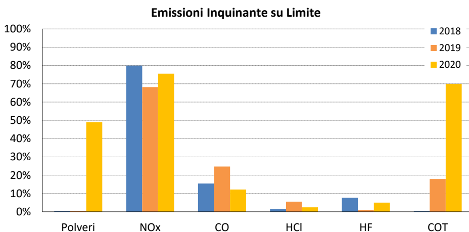
Figura 17 Indicatore "Posizionamento Rispetto al Limite" – E1
