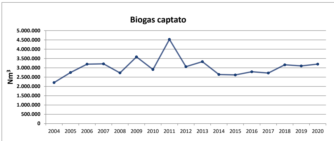
Figura 8 Andamento temporale del quantitativo di biogas estratto dal corpo discarica
