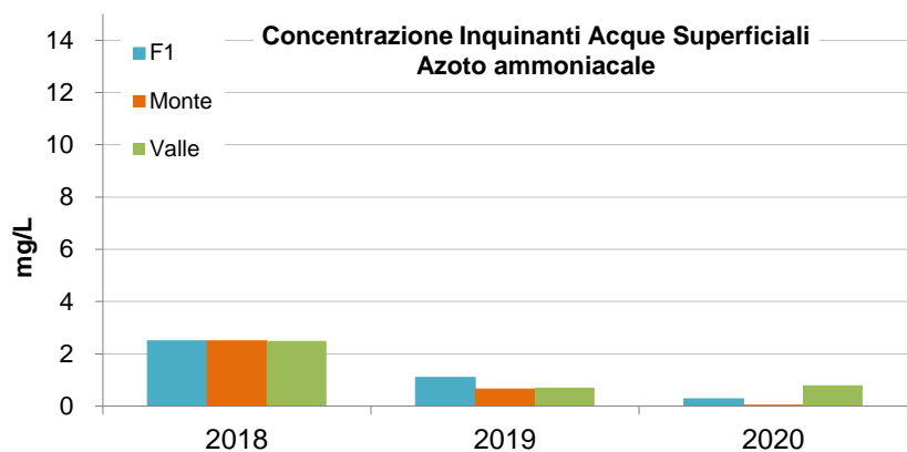
Figura 16 Andamento concentrazione Azoto Ammoniacale triennio 2018-2020
