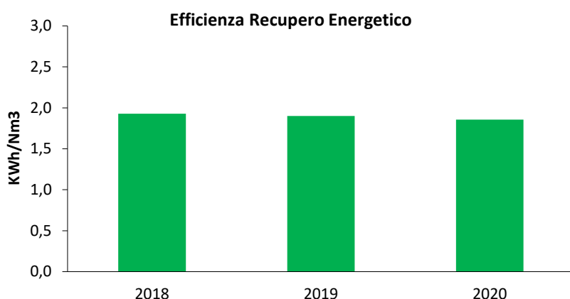
Figura 9 Andamento dell'indicatore "Efficienza di Recupero Energetico"
