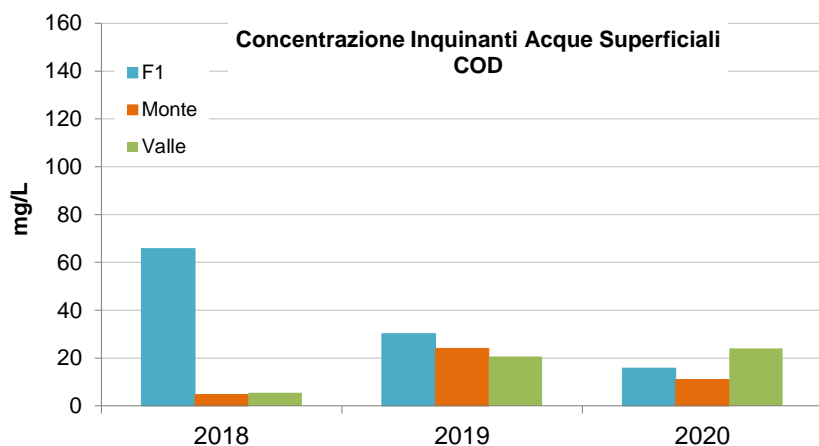
Figura 15 Andamento concentrazione COD triennio 2018-2020
