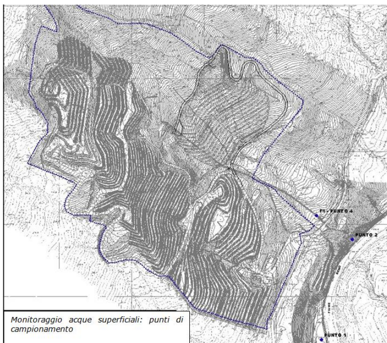
Figura 14 Punti di campionamento
