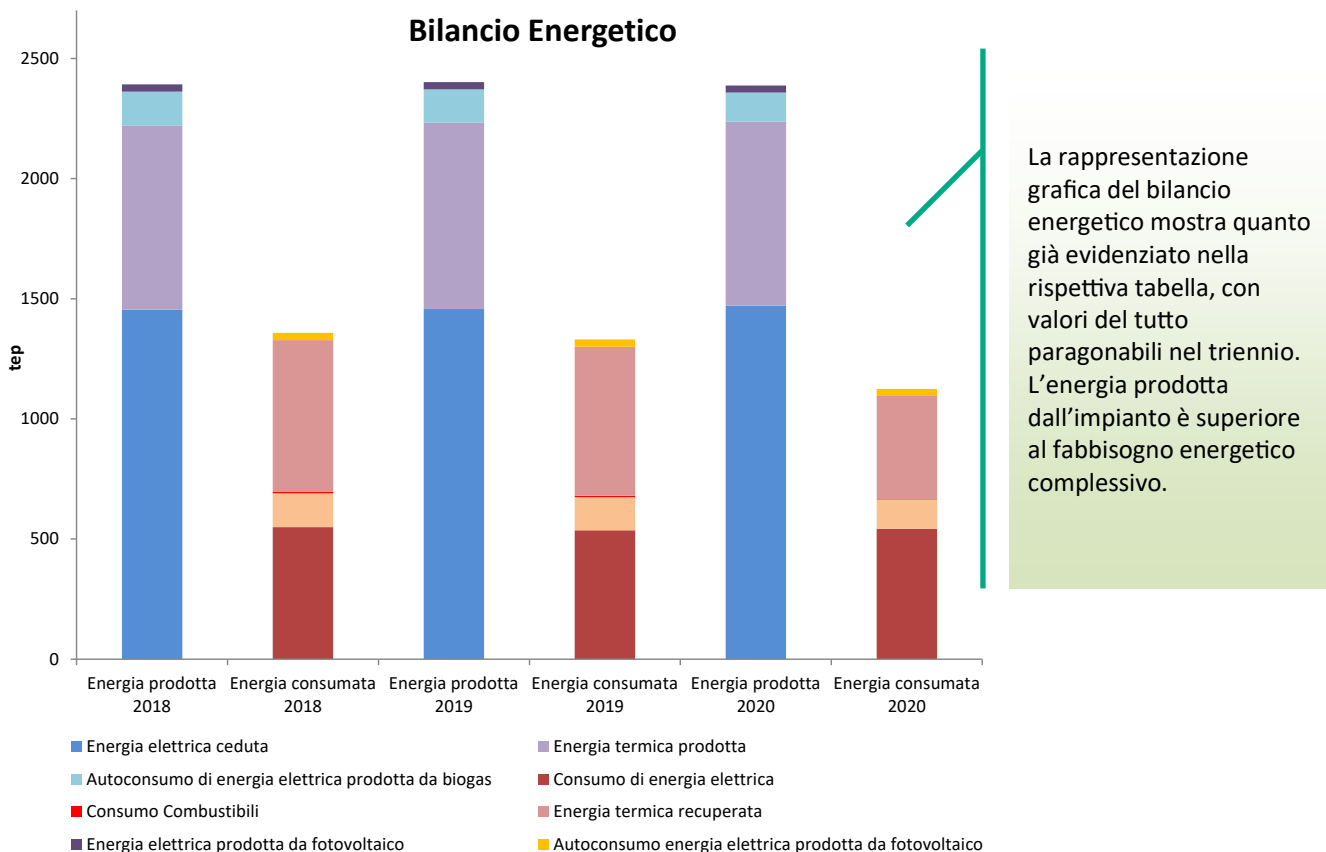
Figura 19 Bilancio energetico dell'impianto di compostaggio
