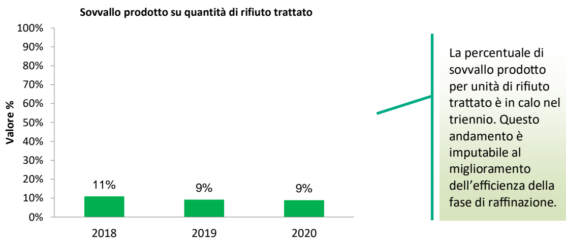
Figura 37 Andamento della produzione di sovrallo in funzione del rifiuto trattato
