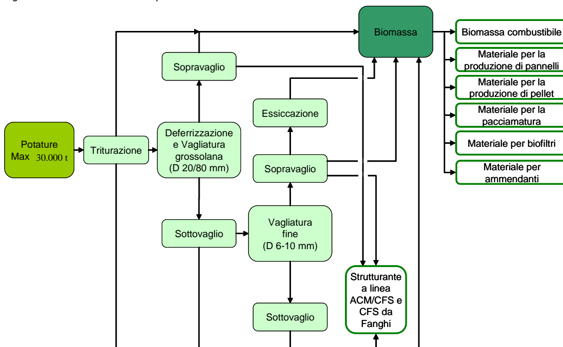
Figura 16 Schema a blocchi del processo
