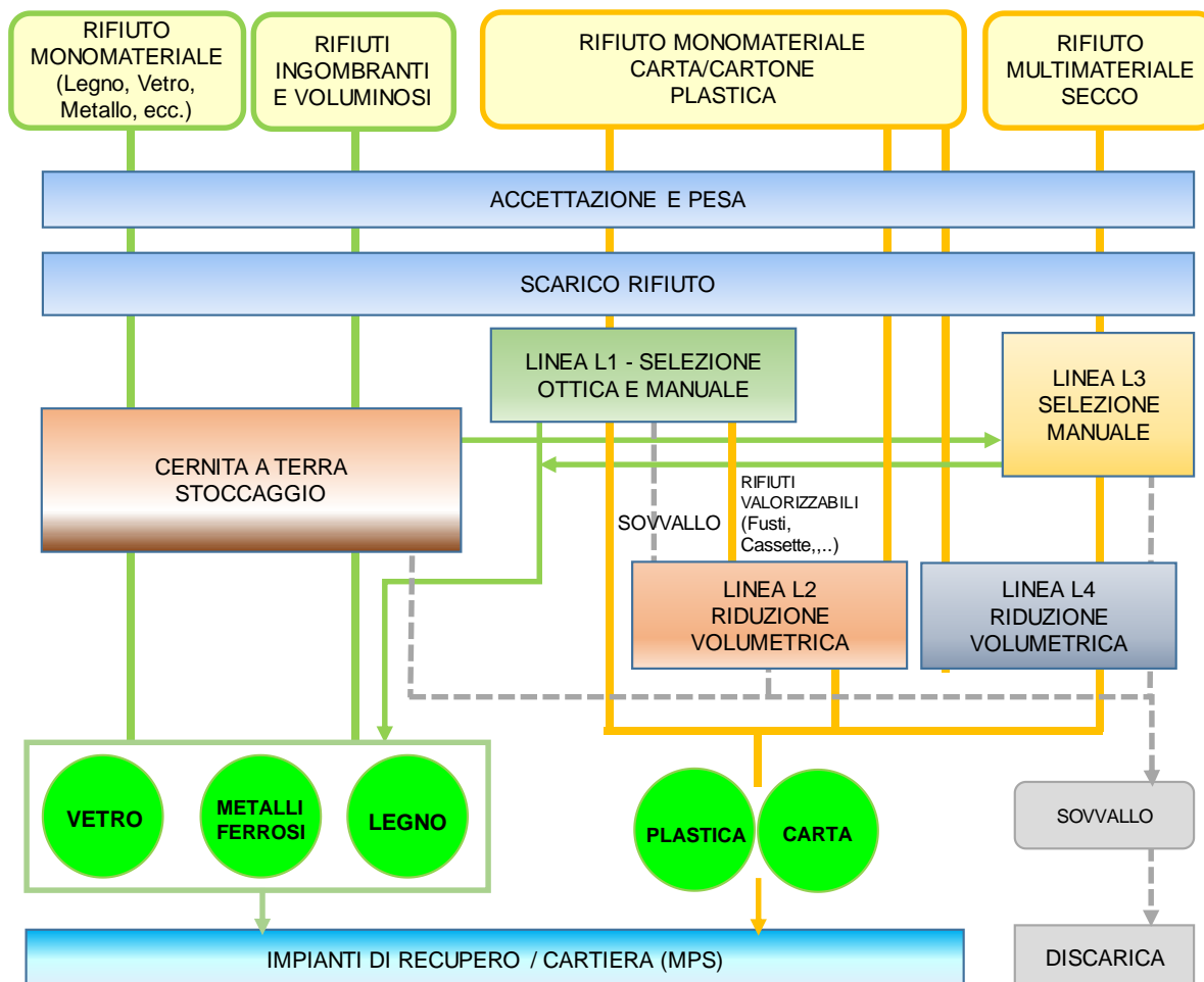
Figura 7 Schema a blocchi delle principali attività del ciclo produttivo
