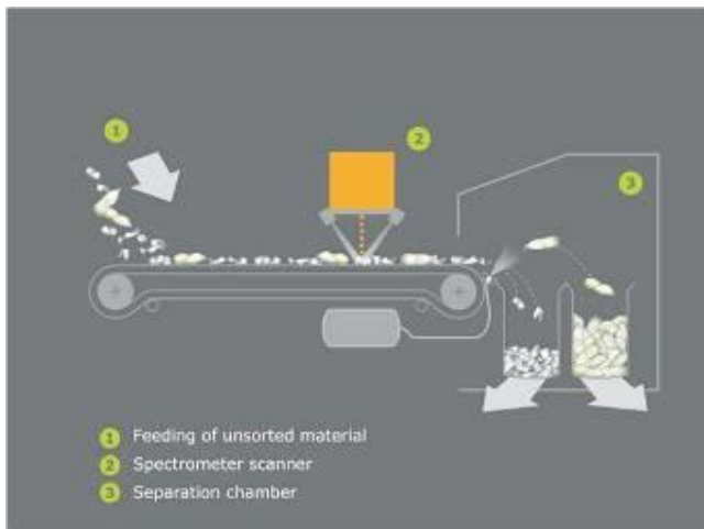
Figura 9 Schema della selezione automatica tramite lettori ottici
