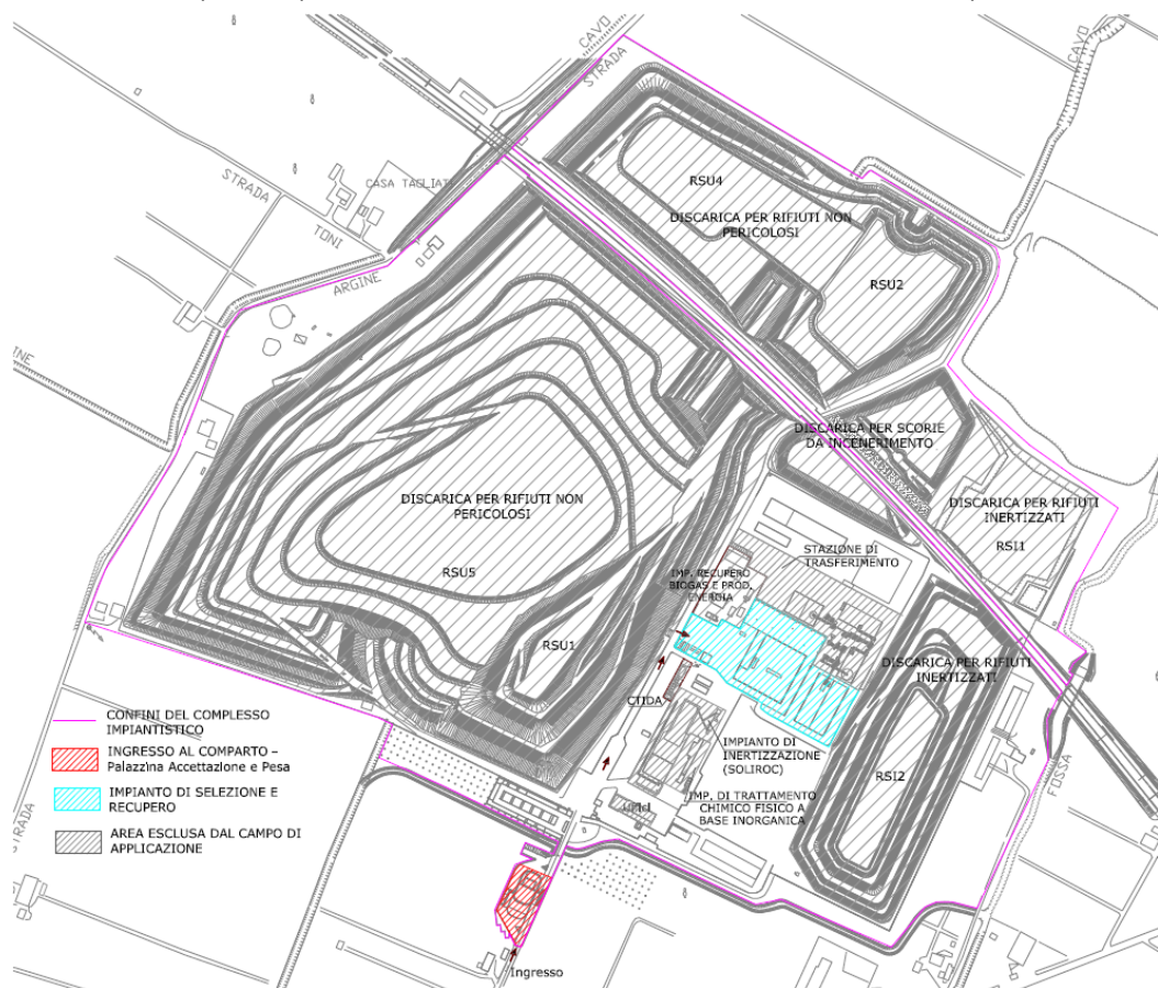
Figura 1 Planimetria del complesso impiantistico di Modena denominato "AREA 3" con le aree di competenza
