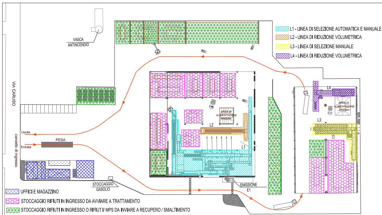
Figura 4 Planimetria del sito
