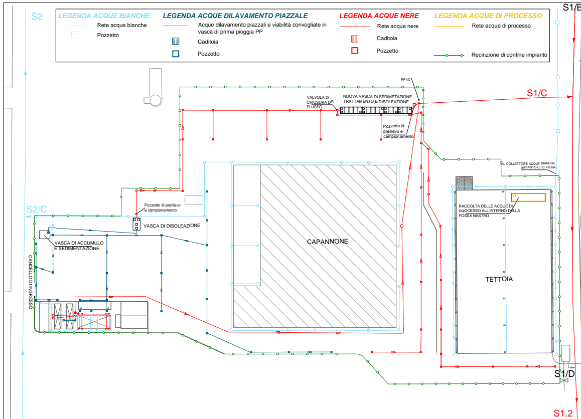
Figura 20 Planimetria degli scarichi idrici
