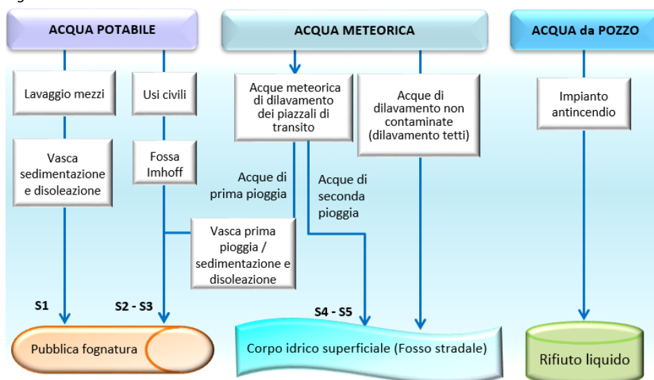
Figura 22 Ciclo idrico
