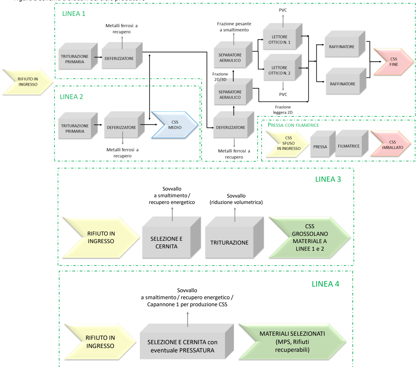
Figura 5 Schema a blocchi del ciclo produttivo
