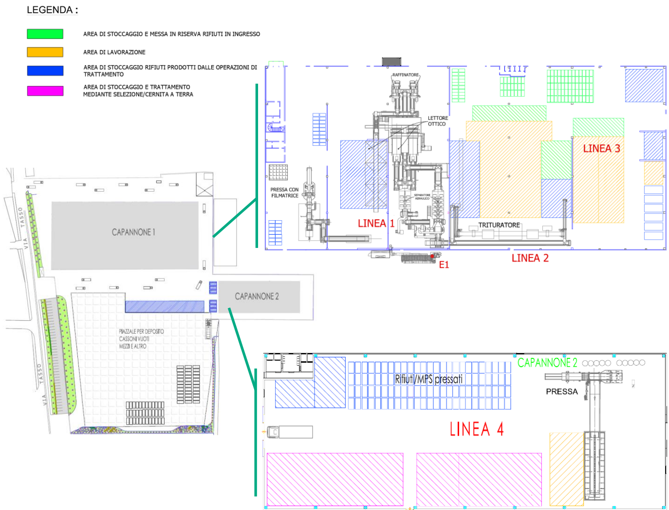
Figura 3 Planimetria del sito
