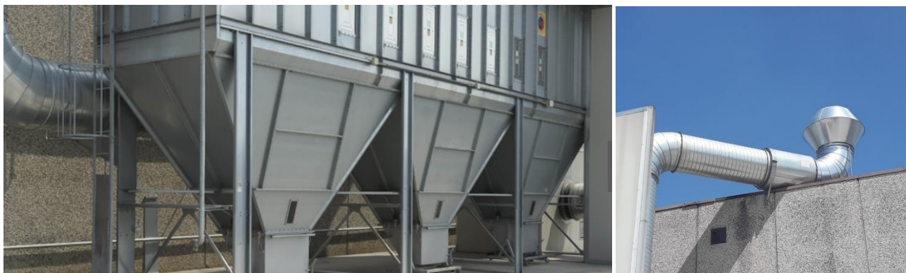
Figura 15 Particolare del filtro a maniche e del punto di emissione
