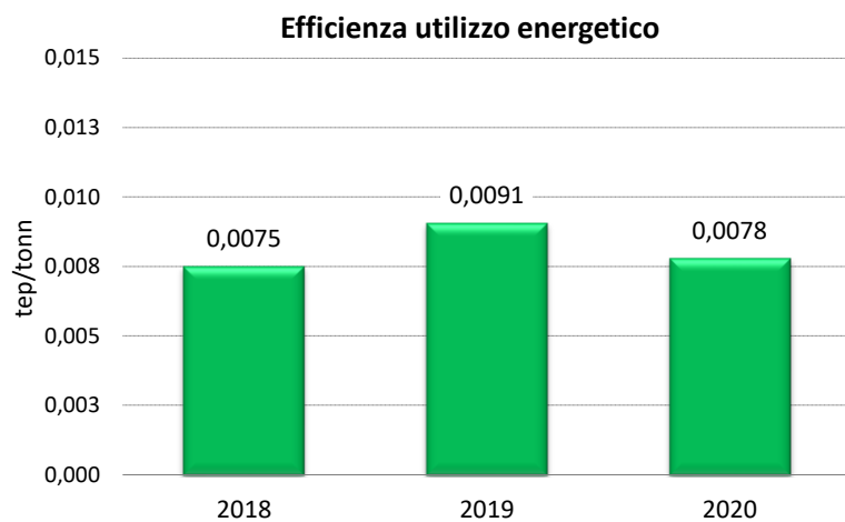
Figura 21 Andamento dell'indicatore "Efficienza di utilizzo energetico"
