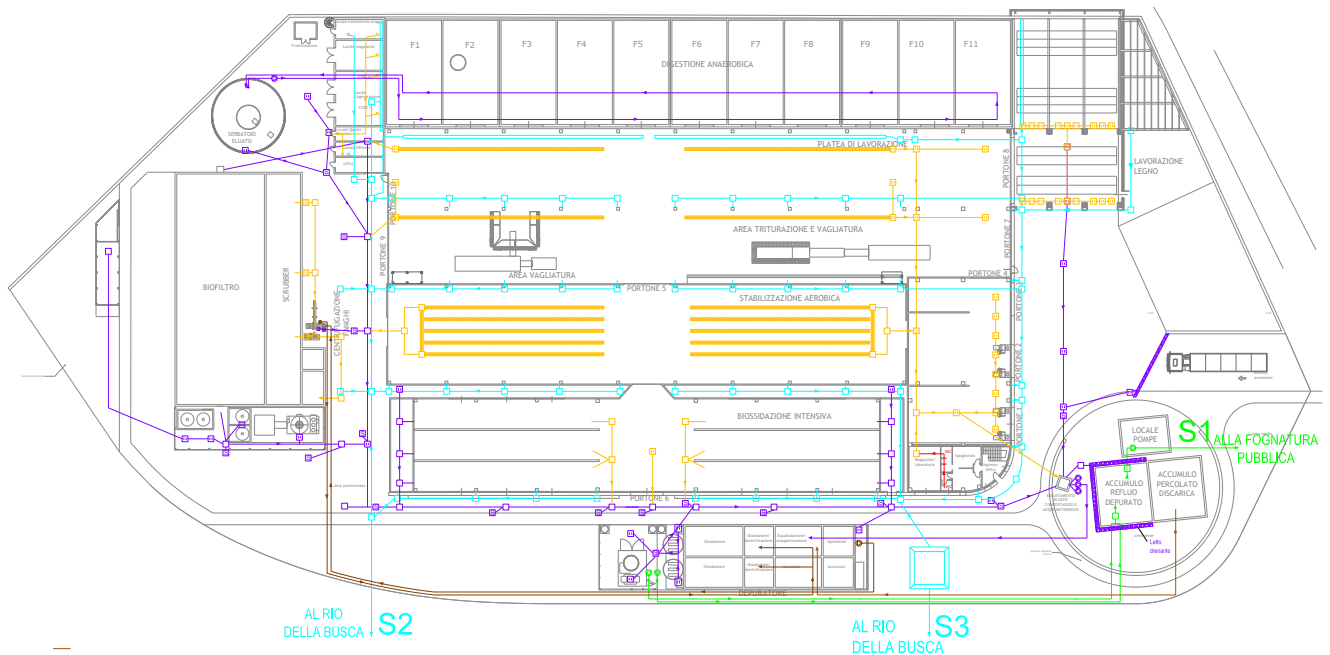
Figura 40 Planimetria degli scarichi idrici
