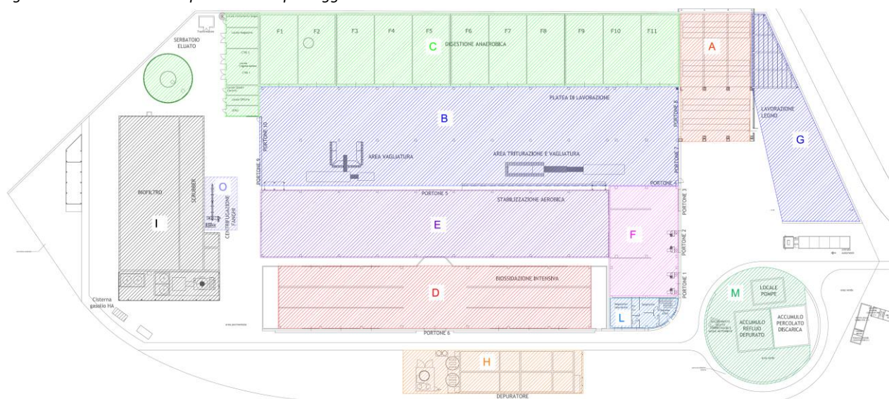
Figura 9 Planimetria dell'impianto di compostaggio
