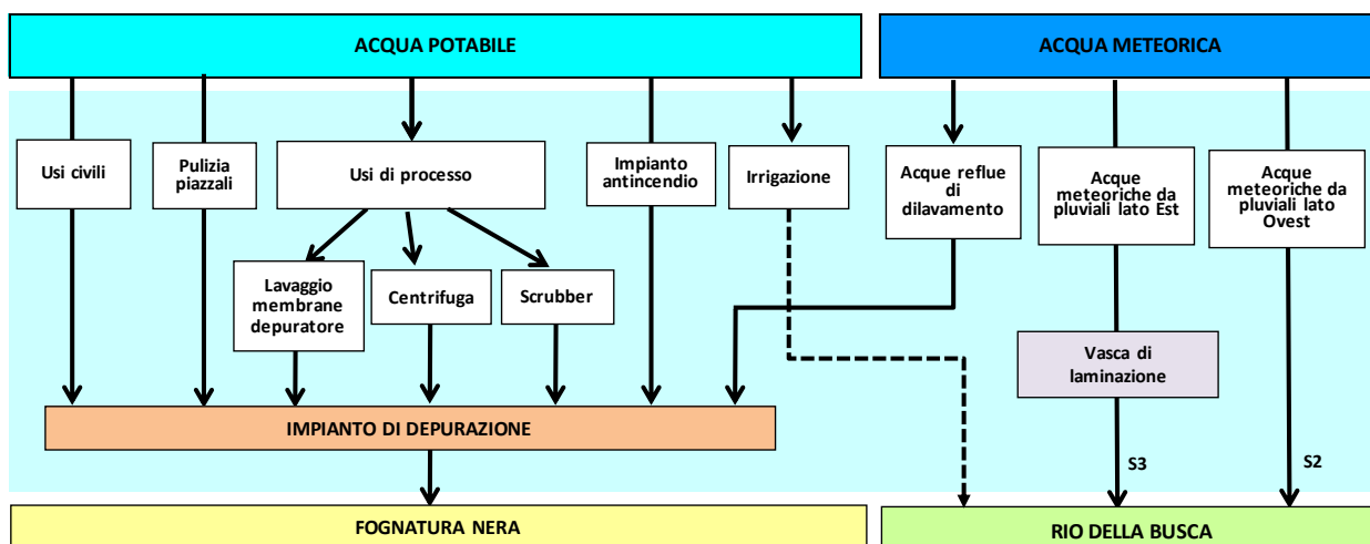
Figura 36 Ciclo idrico
