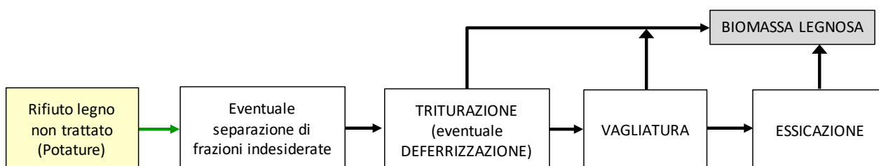
Figura 19 Schema a blocchi del ciclo produttivo
