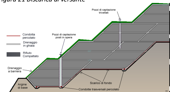
Figura 21 Discarica di versante
