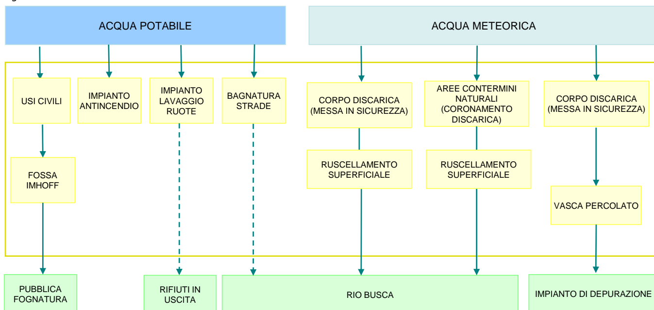
Figura 38 Ciclo idrico
