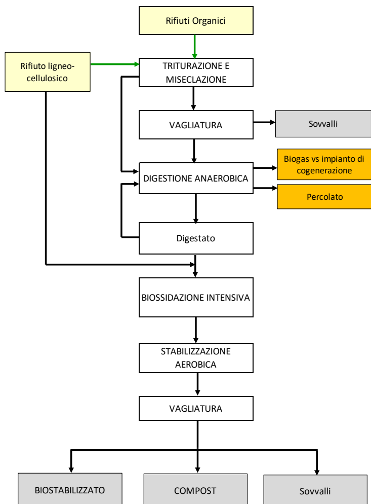
Figura 10 Schema a blocchi del ciclo produttivo
