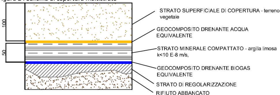
Figura 24 Schema di copertura multistrato
