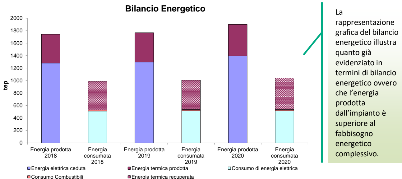
Figura 31 Bilancio energetico dell'impianto di compostaggio
