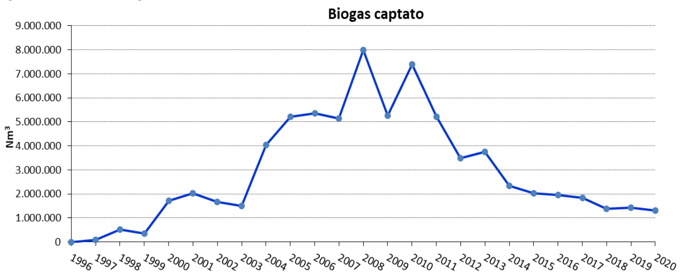
Figura 12 Quantitativi di biogas estratto durante il ciclo di vita della discarica
