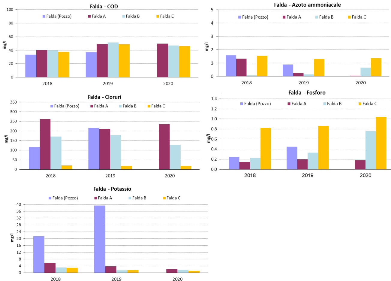
Figura 23 Andamento del COD e dei markers per le acque di falda
