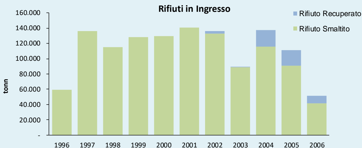
Figura 5 Quantitativi dei rifiuti conferiti durante il ciclo di vita della discarica
