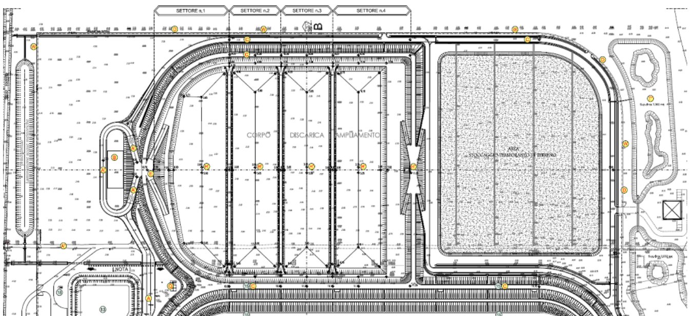
Figura 4 Particolare da progetto nuova discarica
