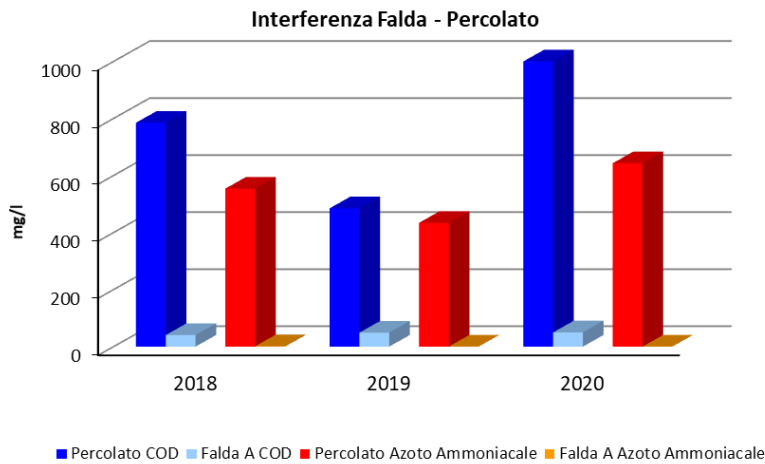
Figura 24 Confronto tra gli andamenti dei markers nel percolato e nella falda A di primo livello
