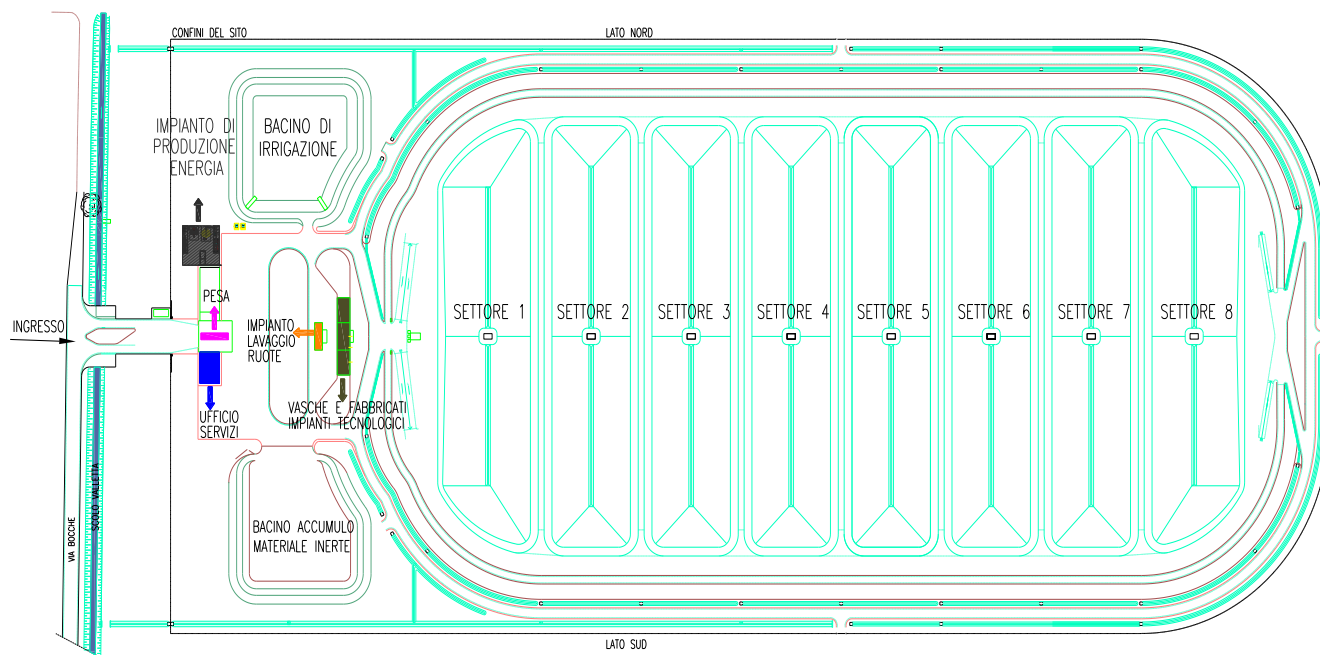
Figura 3 Planimetria del sito
