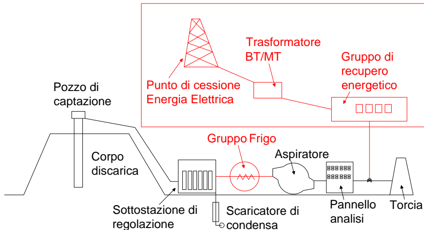
Figura 13 Schema del recupero energetico
