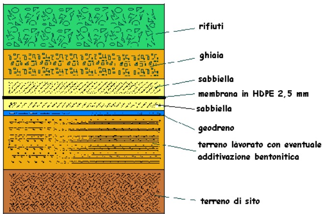
Figura 21 Struttura del fondo della discarica
