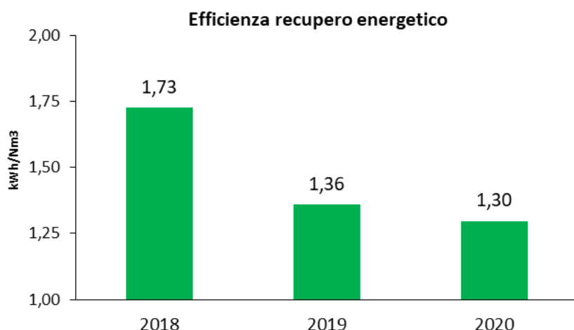
Figura 15 Andamento dell'indicatore "Efficienza di Recupero Energetico"
